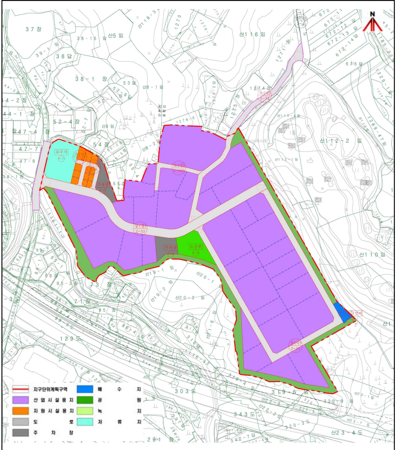
【토지이용계획도】
