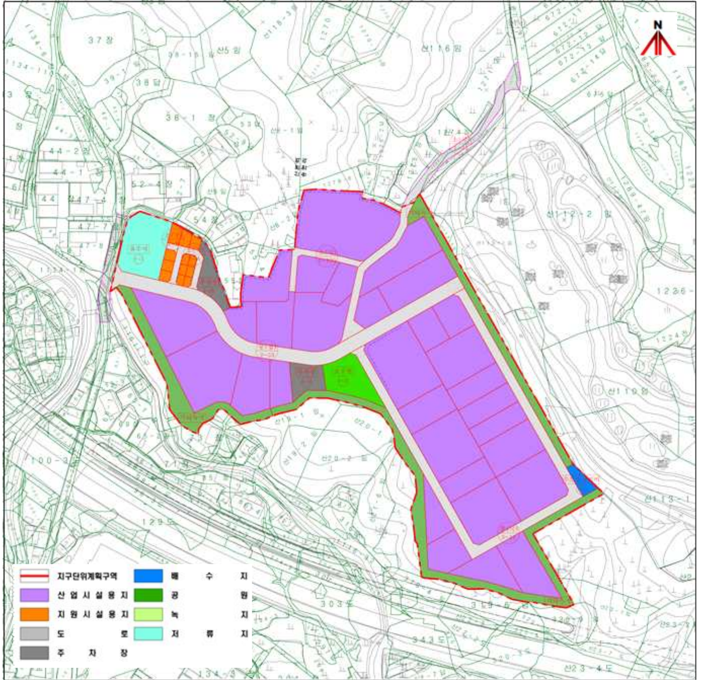
【토지이용계획도】
